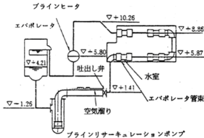
図11 立軸ポンプを負圧満水で棒切始動する場合 [文献(14)抜粋]
